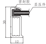
B 短边截面
